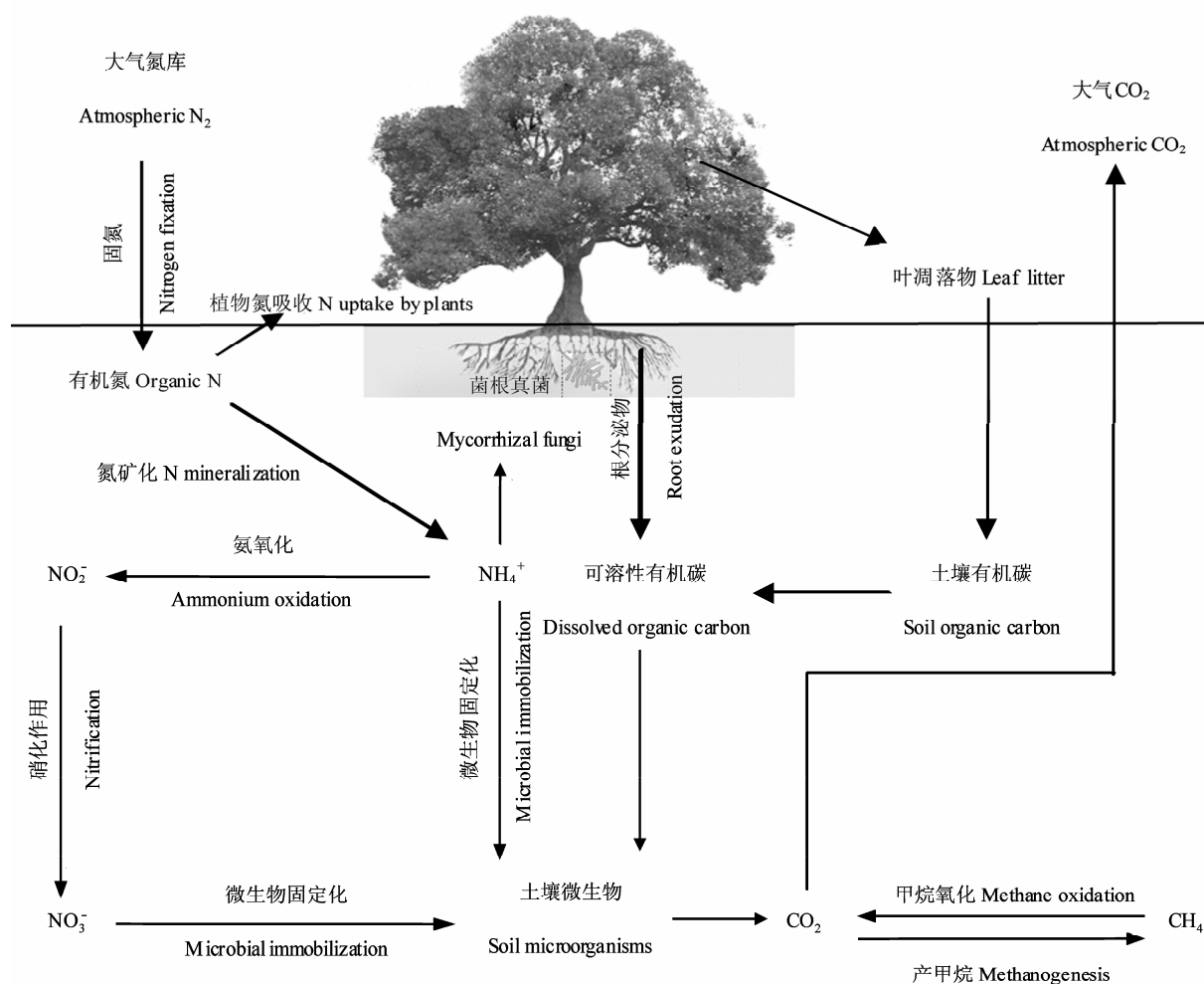
图1 植物与土壤微生物在自然生态系统中的关系(改自Leake et al. , 2004; van der Heijden et al. , 2008)。
